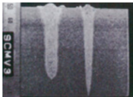
EBWによるシャープな溶込形状
